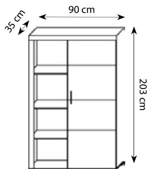
SAMBA witryna wysoka reg. 2
